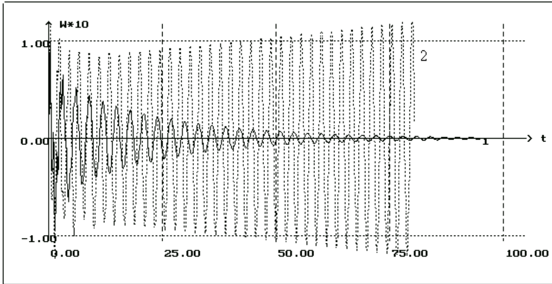
Fig. 7 \lambda_1=180 (1); \lambda_1=240 (2); A=0.1 ; \alpha=0.25 ; \beta=0.05 ; \theta=\pi/6 ; \lambda=1 ; V=510 m/s
