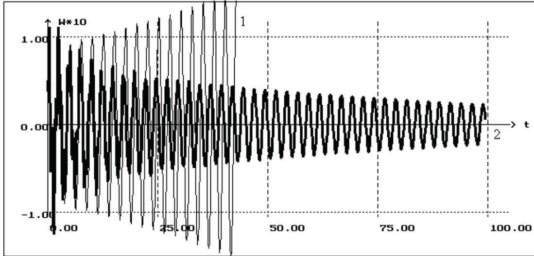
Fig. 5 \alpha=0.1 (1); \alpha=0.4 (2); A=0.1 ; \beta=0.05 ; \theta=\pi/6 ; \lambda=1 ; \lambda_1=220 ; V=510 m/s
