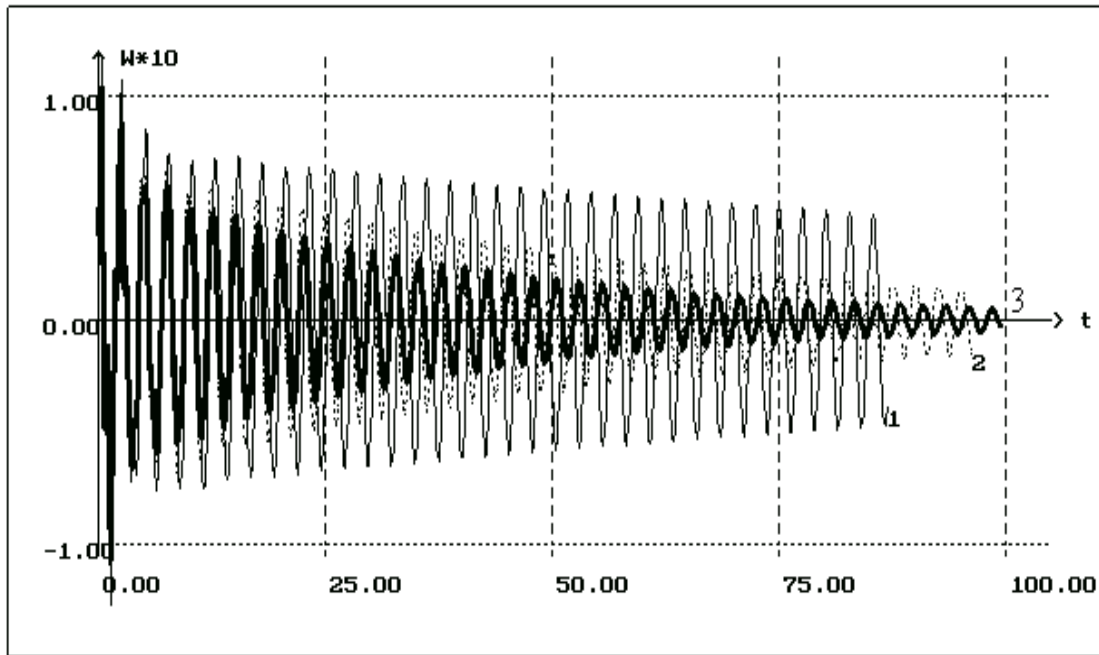
Fig. 6 \theta=0 (1); \theta=\pi/6 (2); \theta=\pi/4 ; A=0.1 ; \alpha=0.25 ; \beta=0.05 ; \lambda=1 ; \lambda_1=220 ; V=510 m/s
