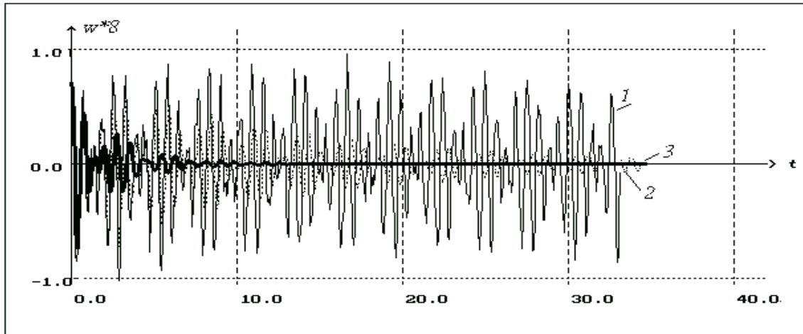
Fig. 4 A=0.001 (1); A=0.02 (2); A=0.1 (3); \alpha=0.25 \beta=0.05 ; \theta=0 ; \lambda=1 ; \lambda_1=220
